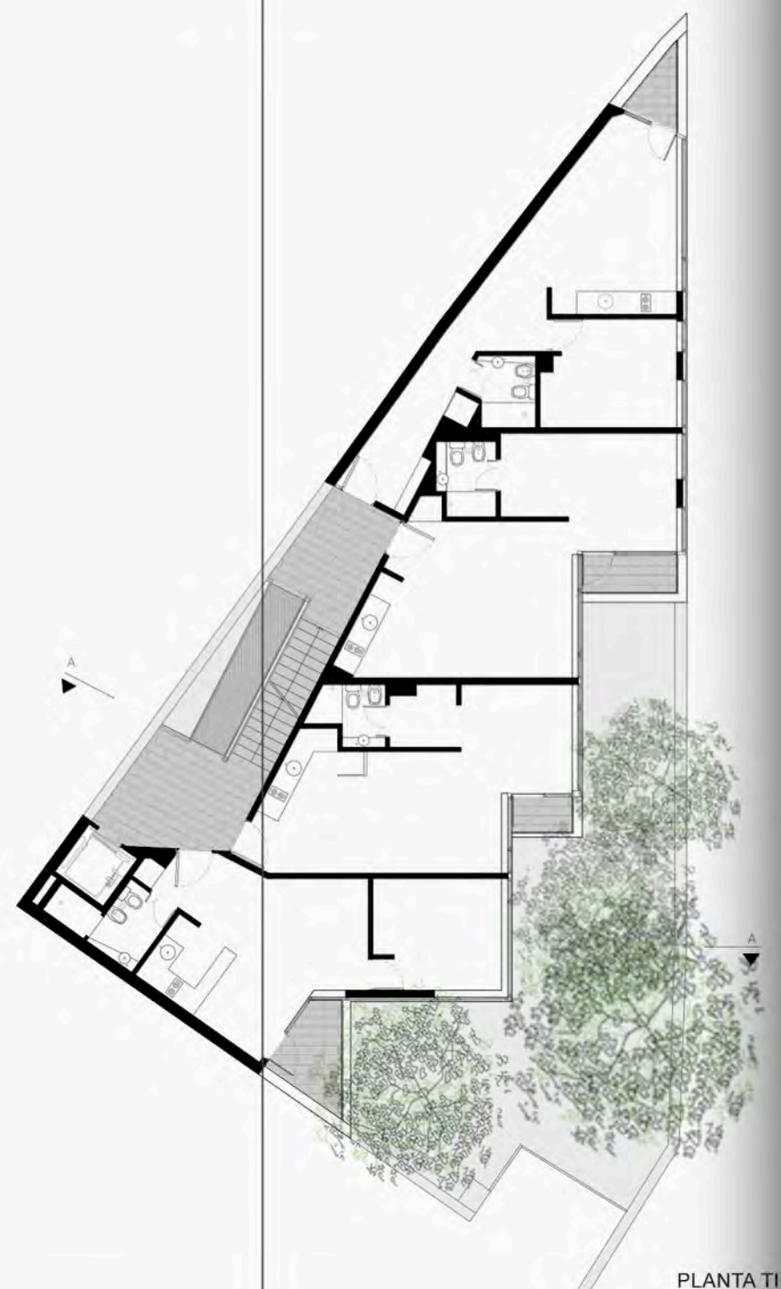
PLANTA TIPO
