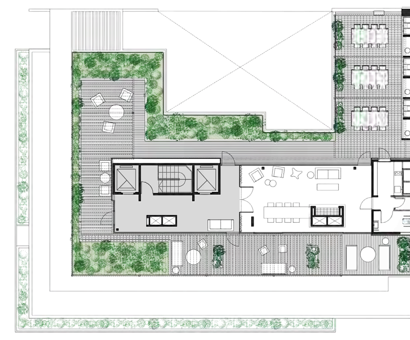
NIVEL 11
